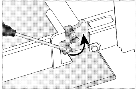
Bloqueio da dobradiça - posição fechada
